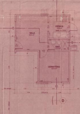
PLANTA-BAIXA CASA TIPO 80-111-01 3 COBERTURAS 27,52 m 2 ESC. 1/50
