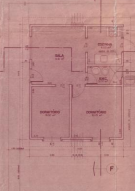
PLANTA-BAIXA CASA TIPO 80-111-02 3 COBERTURAS 34,19 m 2 ESC. 1/50
