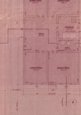
PLANTA-BAIXA CASA TIPO 80-111-04 3 COBERTURAS 43,44 m 2 ESC. 1/50
